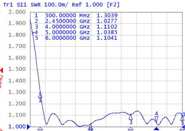
图 2 Input Port VSWR 输入端驻波测试结果
