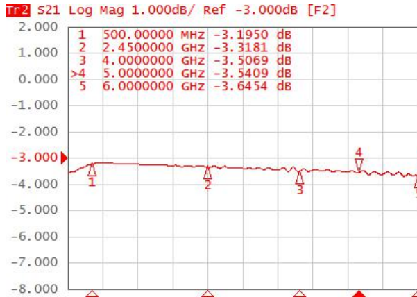
图 1 Insertion Loss 插入损耗测试结果
