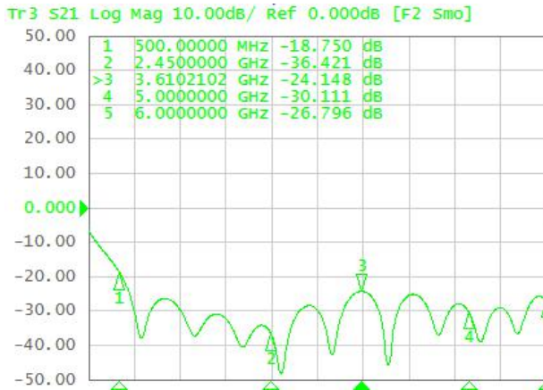
图 3 Isolation 隔离度测试结果
