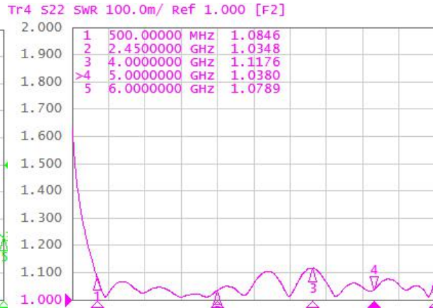
图 4 Output Port VSWR 输出端驻波测试结果
